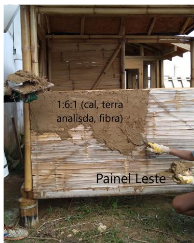
Figuras 11, 12 e 13 – Elaboração, aplicação e texturização do emboço a base de terra estabilizado com cal e fibra
