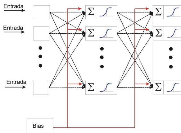
Figura 2: RNA multicamada com camadas de entrada, ocultas e saídas., Fonte: RIBEIRO, 2003
