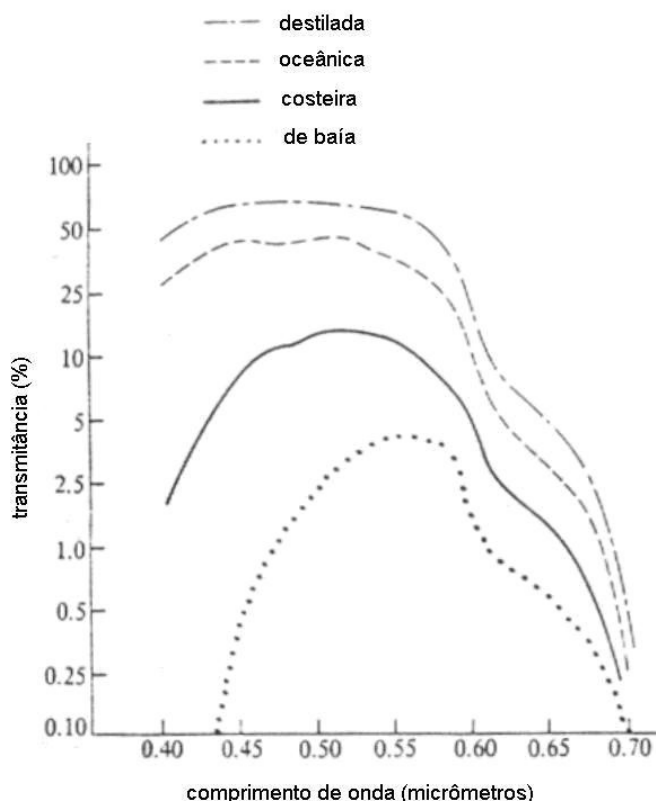
Figura 1: Curva de transmitância da água, Fonte: SWAIN e DAVIS, 1978.
