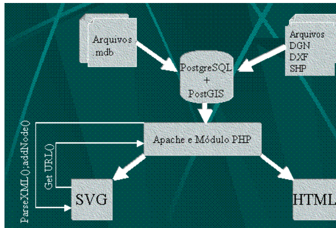
Figura 6 : Fluxograma representando as etapas de desenvolvimento do trabalho
