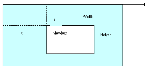
Figura 3 : Visão da viewBox em SVG
