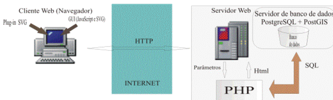
Figura 4 : Esquema da arquitetura Cliente/Servidor em três camadas a ser adotada
