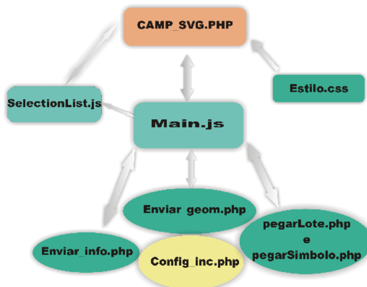
Figura 7 : Esquema de relacionamento entre os códigos implementados
