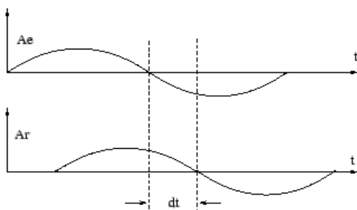
Fig. 2 : Princípio de medição de tempo no sistema de onda contínua
